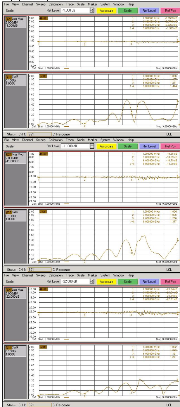
Графики для АЧХ - Log Mag, при отсчётном уровне равном -1 дБ, и для КСВ - SWR
