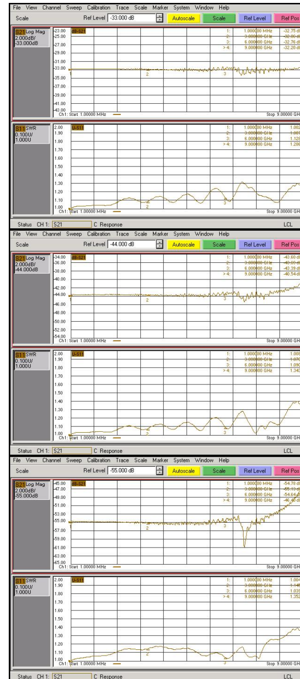
Графики для АЧХ - Log Mag, при отсчётном уровне равном -33 дБ, и для КСВ - SWR
