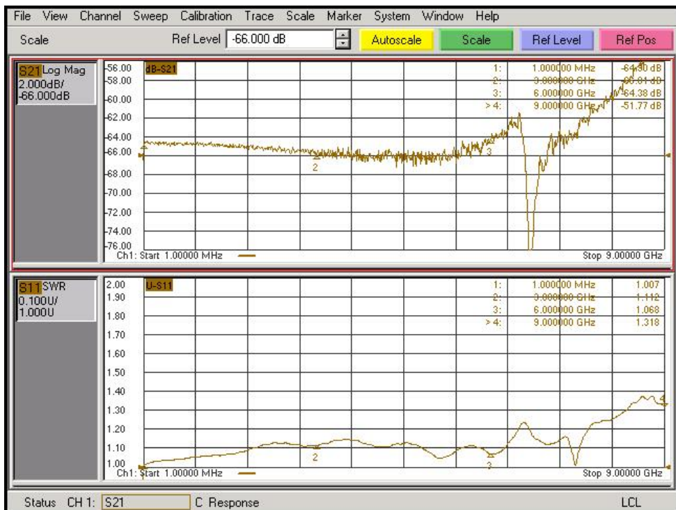
Графики для АЧХ - Log Mag, при отсчётном уровне равном -66 дБ, и для КСВ – SWR
