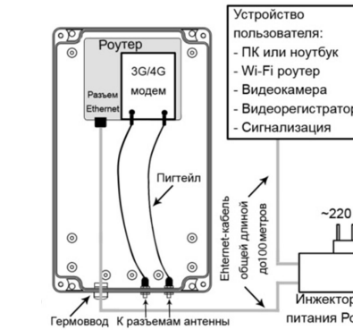
Пример размещения оборудования в гермобоксе
