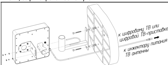
Рисунок 2 – Монтаж антенны на стеновом кронштейне
