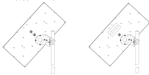
Рисунок 3 – X-поляризация
